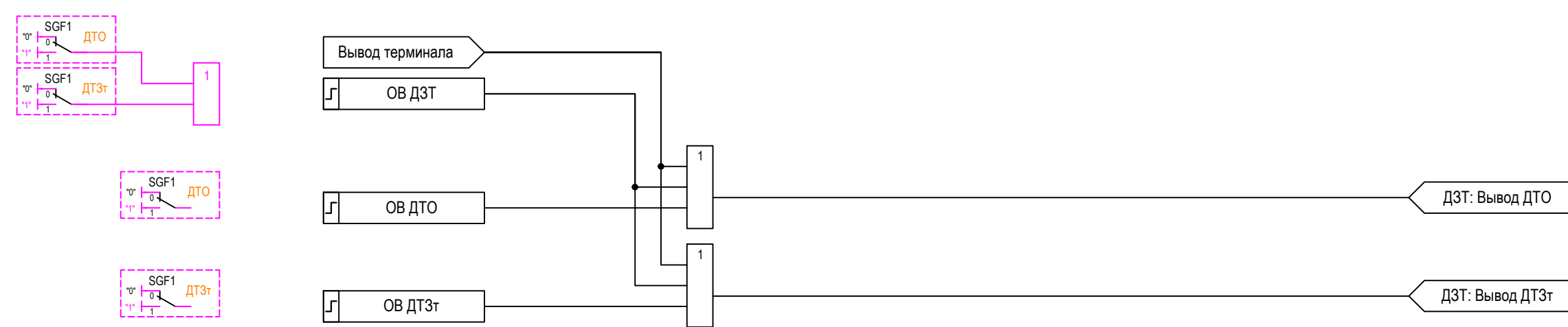
Дифференциальная токовая отсечка (ДТО) (INSPDIF)
