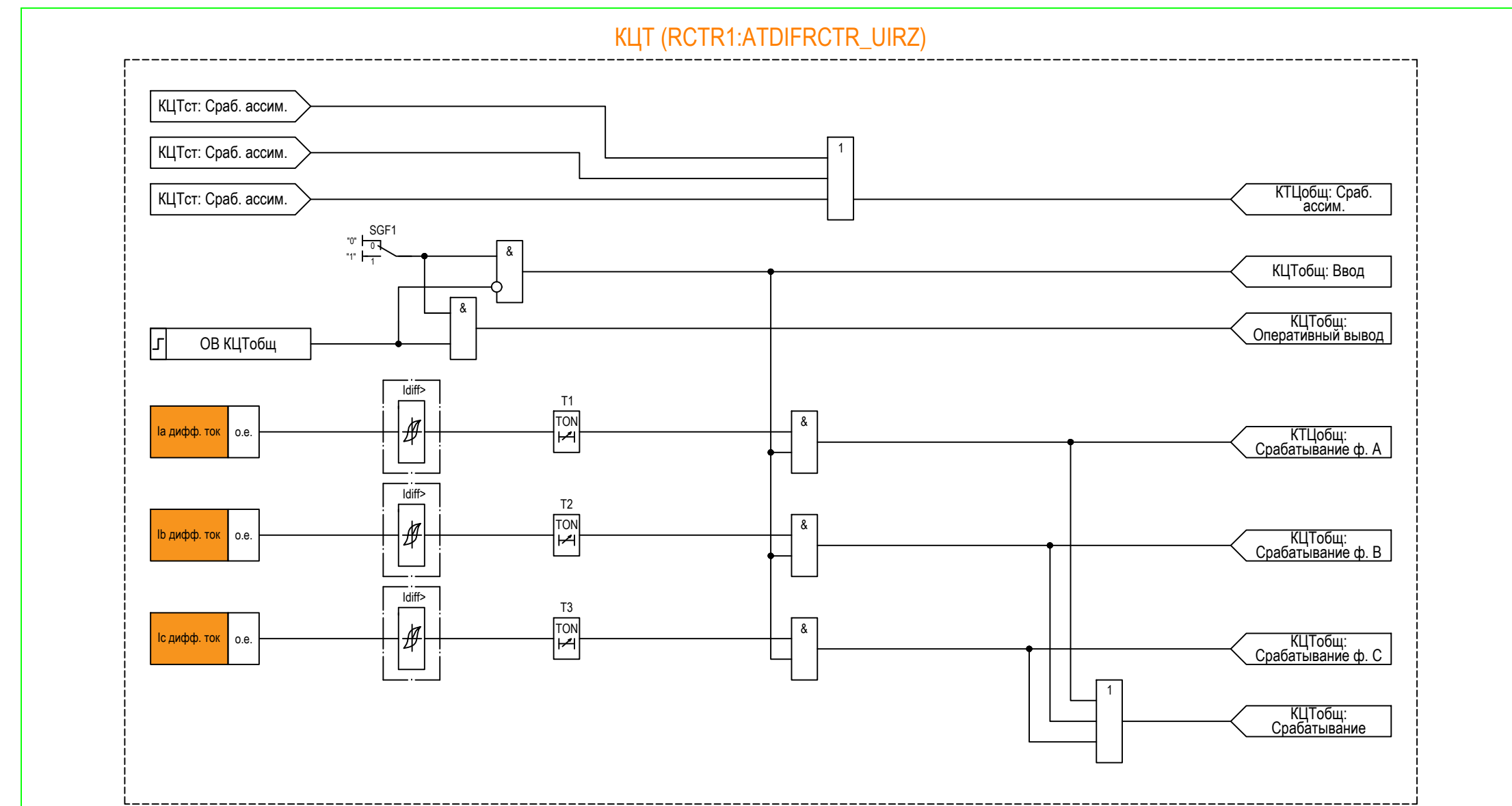
ИО КЦТ - контроль исправности токовых цепей RCTR1:ATDIFRCTR_UIRZ)
