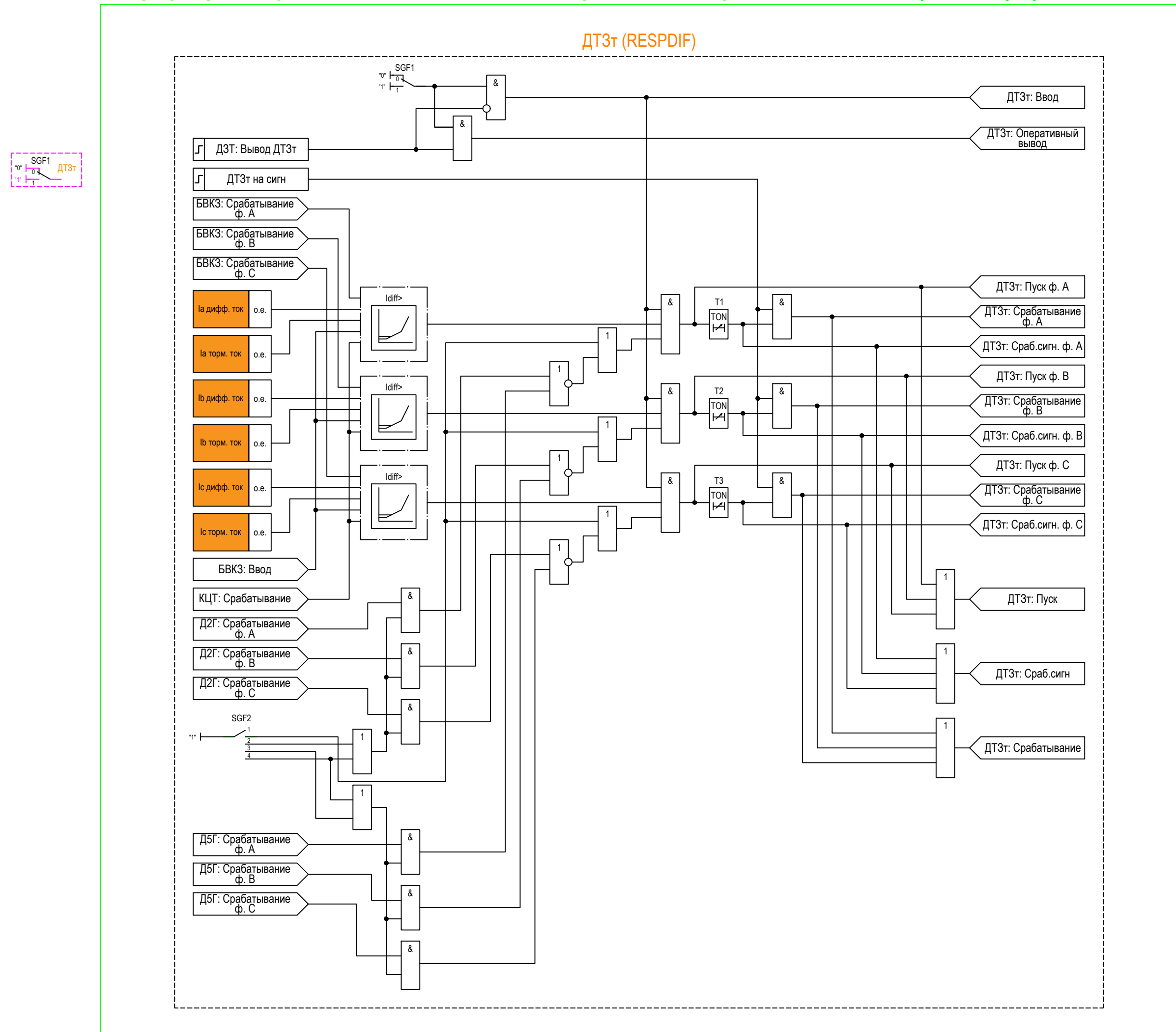
Дифференциальная токовый орган с торможением (ДТЗт) (RESPDIF)
