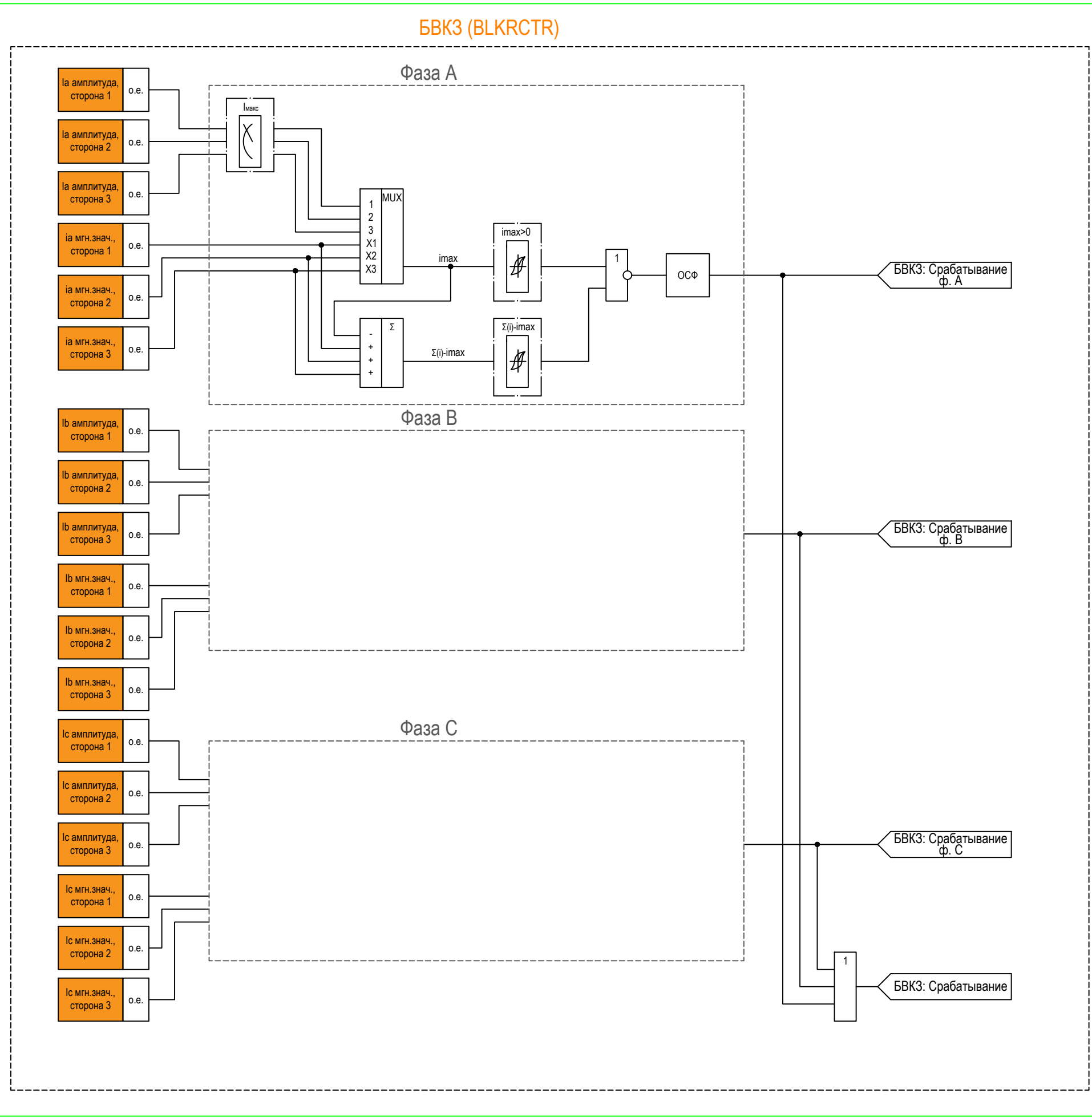
ИО БВКЗ - блокировка при внешних КЗ (BLKRCTR)
